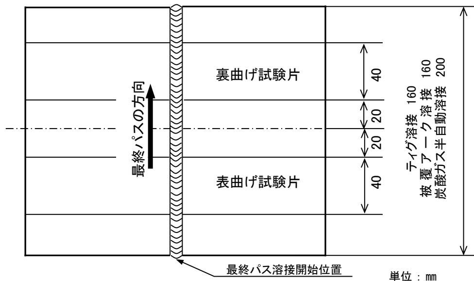
図3 曲げ試験片の採取位置(第一部・第二部を除く)
