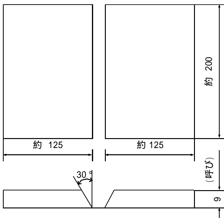
[図 9] 下向中板 (単位 : mm) : [S N - 2 F 相当]
